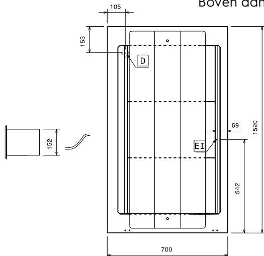
Boven aanzicht
