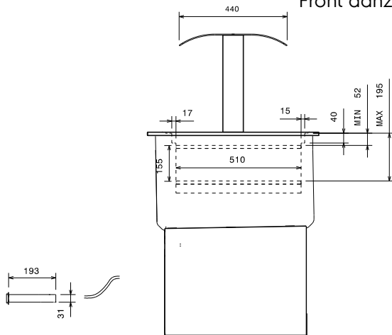
Front aanzicht
